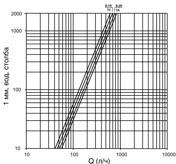
Однотрубный режим
