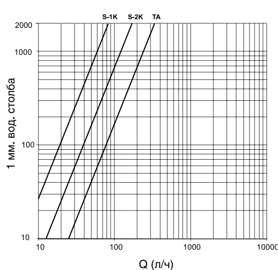
Двухтрубный режим
