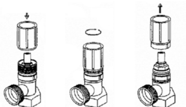
4) Наденьте обратно ручку и затягивайте до момента снятия муфты с корпуса вентиля
