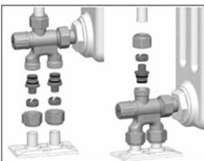
Пример установки с использованием концевок (код 6052) для труб РЕХ.
