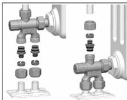
Пример установки с использованием концевок (код 6055) для металлопласт. труб.
