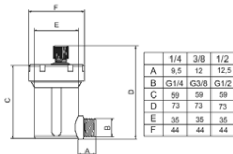
Угловой воздухоотводчик
