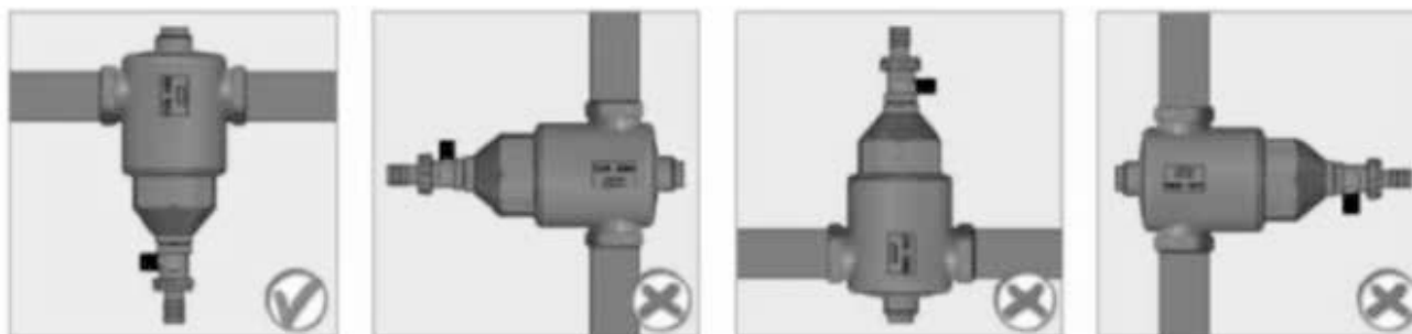
Правильная установка
